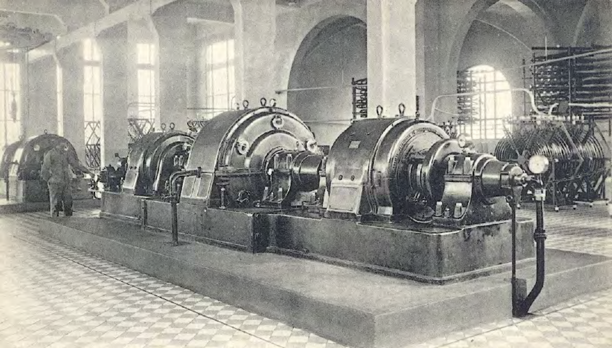
Compagnie RADIO-FRANCE. — Centre de T. S. F. de Sainte-Assise. Station Transcontinentale — Vue d'ensemble d'un groupe alternateur à haute fréquence de 500 kws.
