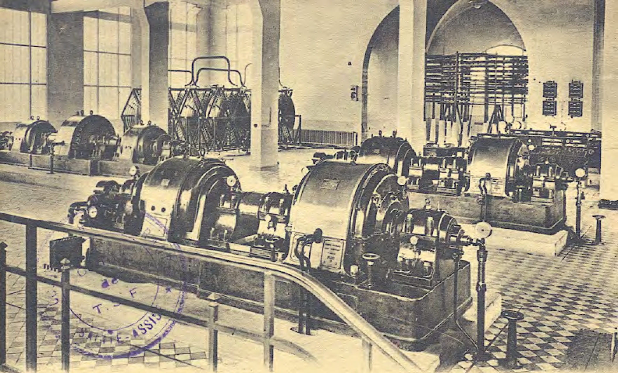
Un coin de la Salle d'émission
