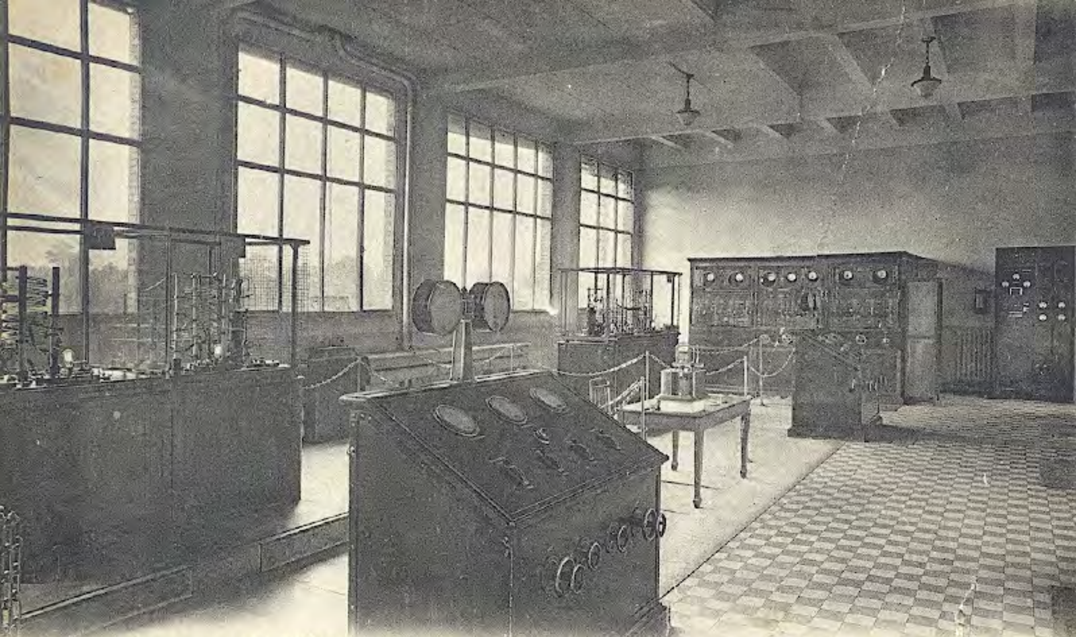
3) Compagnie RADIO-FRANCE. — Centre d'Emission de T. S. F. de SAINTE-ASSISE Vue intérieure d'une Station à Ondes Courtes, type dit à autogénération.
