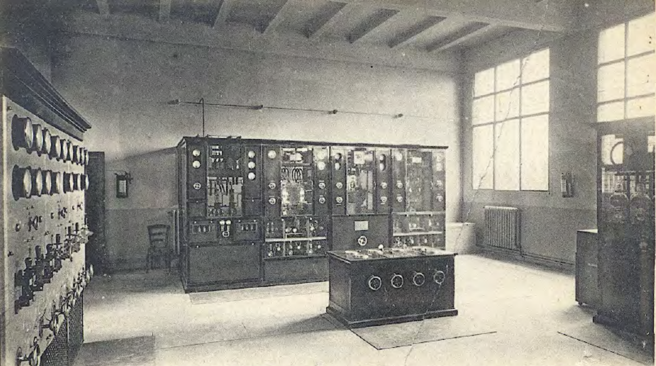
Compagnie RADIO-FRANCE. — Centre d'Emission de T. S. F. de SAINTE-ASSISE Vue intérieure d'une Station à Ondes Courtes, type stabilisé par quartz.
